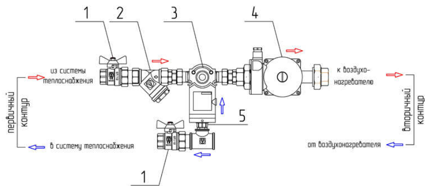
Рисунок 2. Схема смесительного узла
